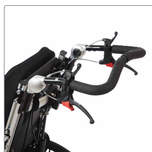
Skubbebøjle med knækfunktion kan ved hjælp af værktøj højdejusteres
