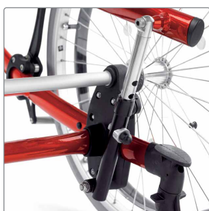
Højdejustering af sæde bagtil på sæderammen
