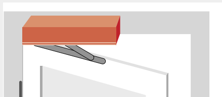
Karmmontage med glideskinne arm
