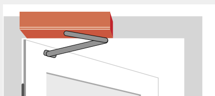
Karmmontage med normal arm
