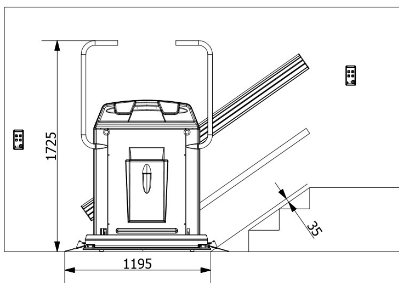
FASTMONTERET BETJENING TIL INDBYGNING ENTEN I SØJLE ELLER MURVÆRK.
