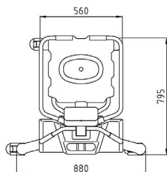
Stollift (mål i mm)
